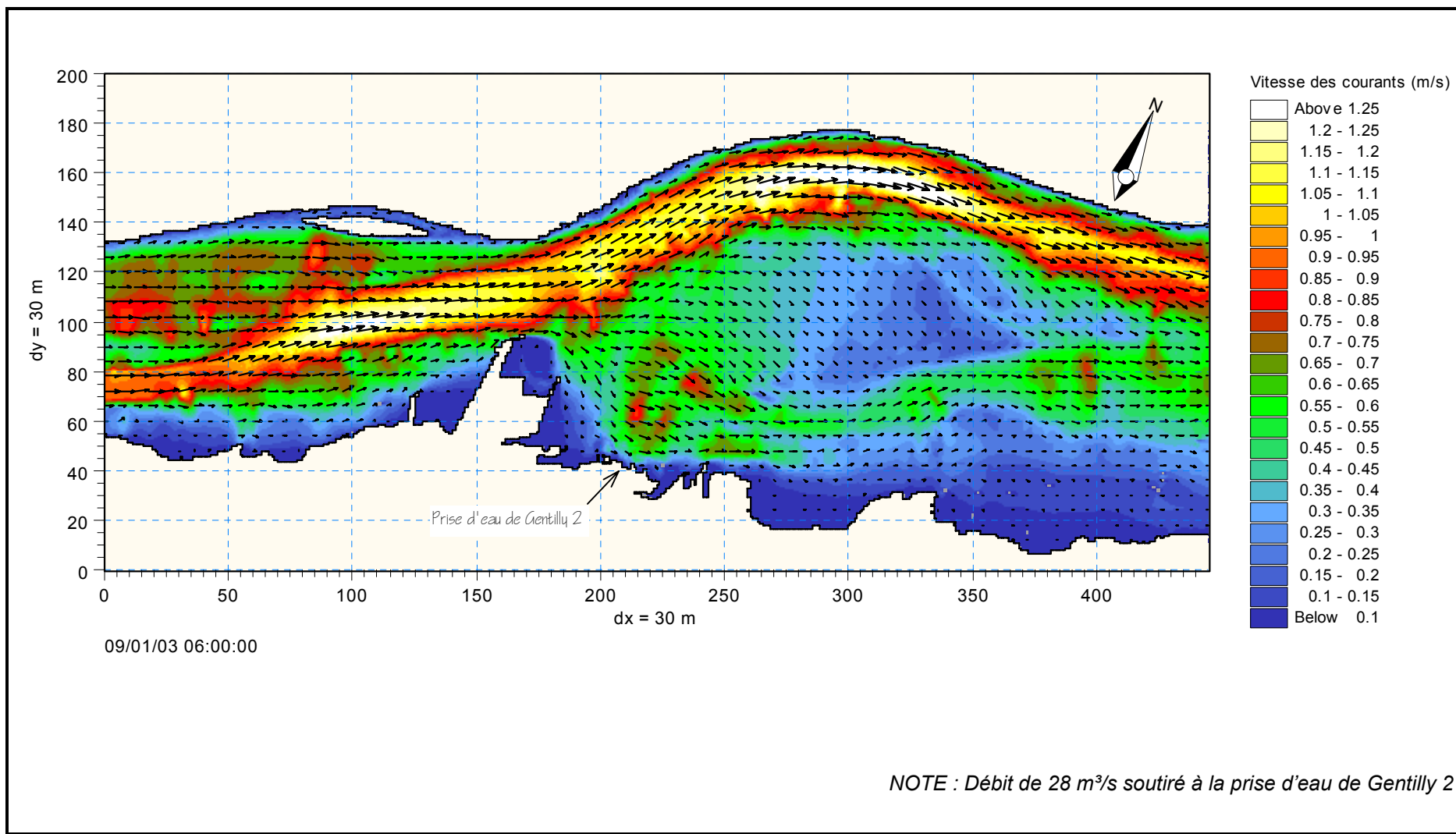
Figure 2.7 Champs de vitesse du fleuve – débit moyen
